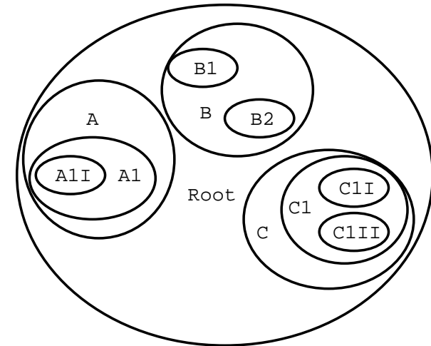
Abbildung 7.2: Baumdarstellung als Summe von Mengen
