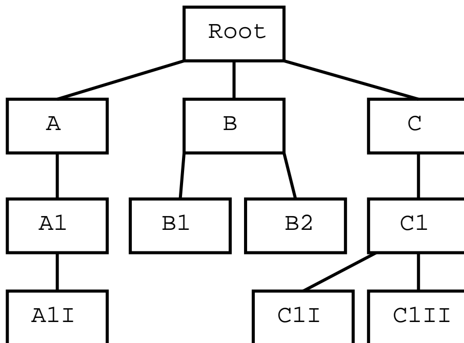
Abbildung 7.1: Unser Baum-Beispiel
