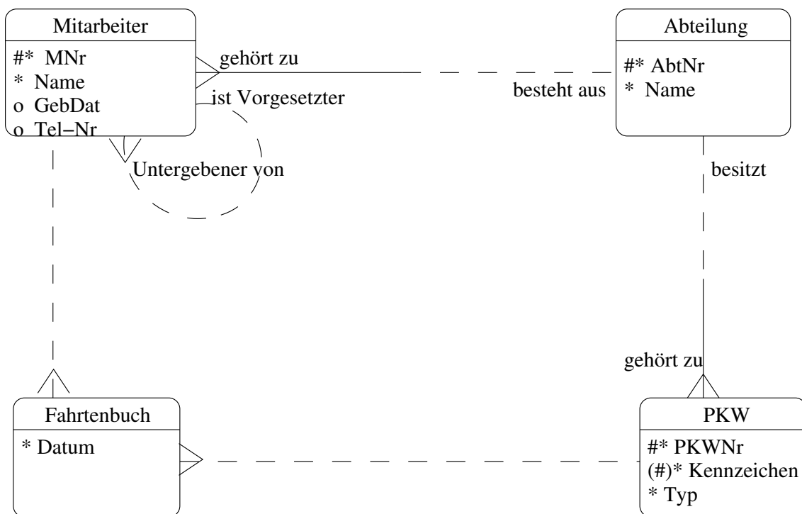
Abbildung 4.3: ER-Beispiel 2
