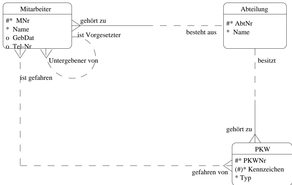
Abbildung 4.2: ER-Beispiel 1
